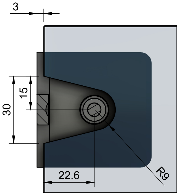
Glas med fräsning
