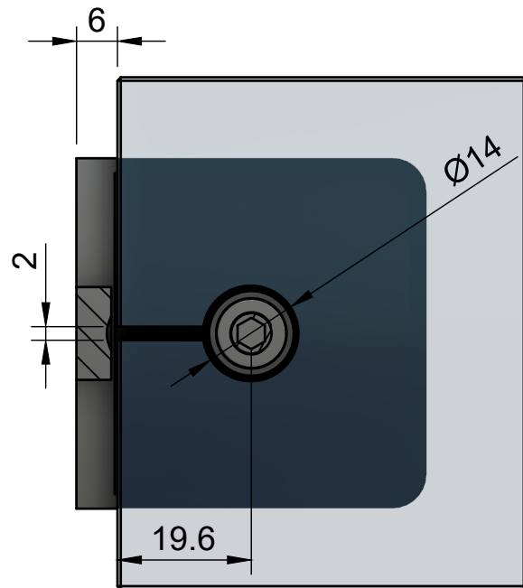
Glas med Ø14 hål och tekniskt snitt
